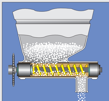
Conjunto para algodão com linter
